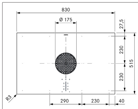
Afb. 3.4 PUX2/R toestelafmetingen bovenaanzicht
