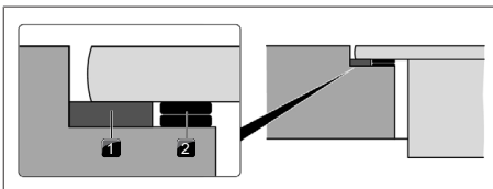
Afb. 11.22 Vulplaatjes
