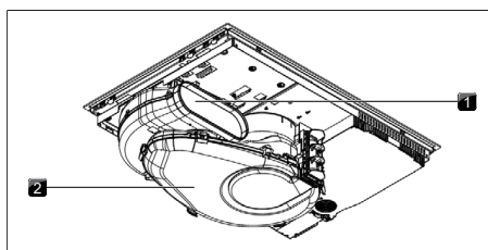
Afb. 4.2 Achteraanzicht luchtafvoervariant
