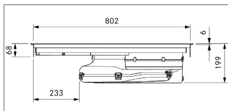
Afb. 3.5 PUX2/R toestelafmetingen vooraanzicht
