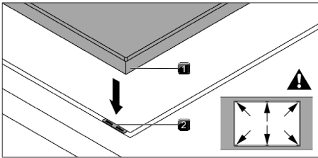
Afb. 11.21 Positionering van de vulplaatjes
