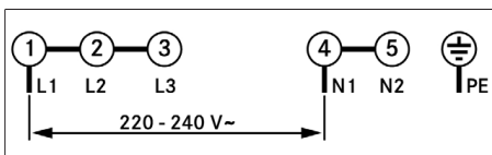
Afb. 11.28 Aansluitschema 1-faseaansluiting
