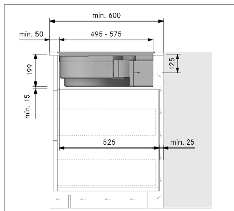
Afb. 11.16 Inbouwmaten bij recirculatie - montagevariant B, werkbladdiepte 600 mm
