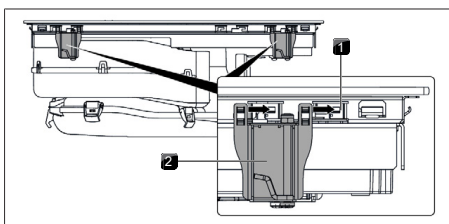
Afb. 11.19 Montageklemmen aanbrengen
