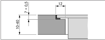
Afb. 11.6 Voegmaat voor vlinkinbouw
