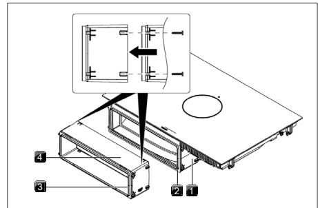
Afb. 11.15 Verlenging telescopisch kanaal
