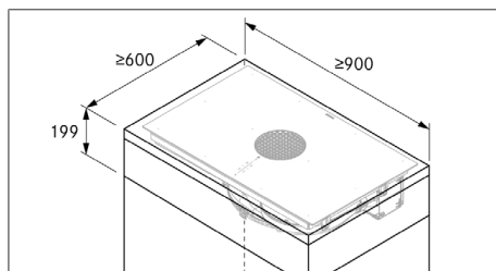
Afb. 11.4 Minimale meubelafmetingen X Pure
