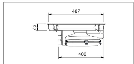
Afb. 3.3 PUXA2/R toestelafmetingen zijaanzicht
