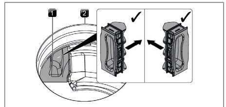
Afb. 9.10 Filtervervangingsklep plaatsen
