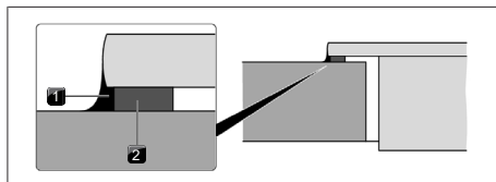
Afb. 11.17 Afdichtingsband bij opbouwmontage
