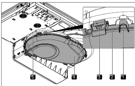
Afb. 9.3 Luchtgeleidingsbehuizing
