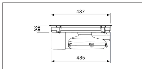
Afb. 3.6 PUX2/R toestelafmetingen zijaanzicht
