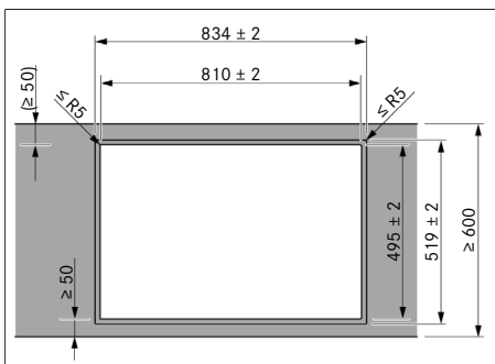
Afb. 11.5 Uitsparingsafmetingen in geval van vlakinbouw
