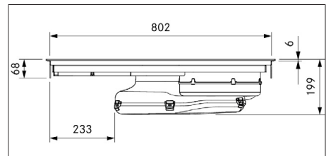
Afb. 3.2 PUXA2/R toestelafmetingen vooraanzicht
